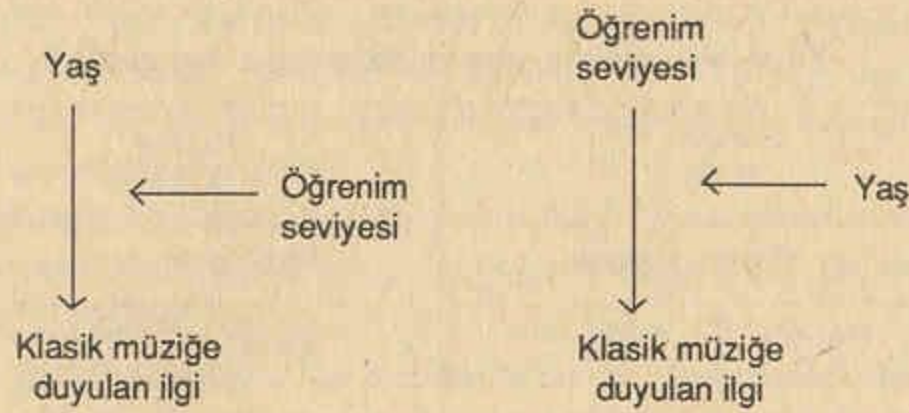
Şekil 5. Tablo VI'ya denk düşen nedensel yapılar.
