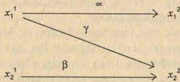
Şekil 6. Tablo VI'nın verilerine denk düşen yapı.
