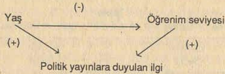
Şekil 4. Tablo V'e denk düşen nedensel yapı.
