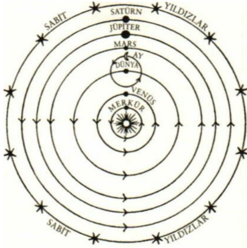
Kopernik'in Evren'i.
