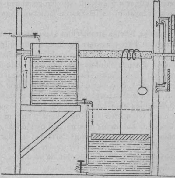
Şekil 9 - F.Maitzinger tarafından tasarlanmış büyük sarkaç denemesi Bu tip sarkaç Roma İmparatorluk döneminde birçok bölgede kullanılmış olmalıdır. Sarkacın amacı köleleri uyandırmak ve onların verimini ölçmektir. (Tardy, La Pendule Française (Fransız Sarkacı))
